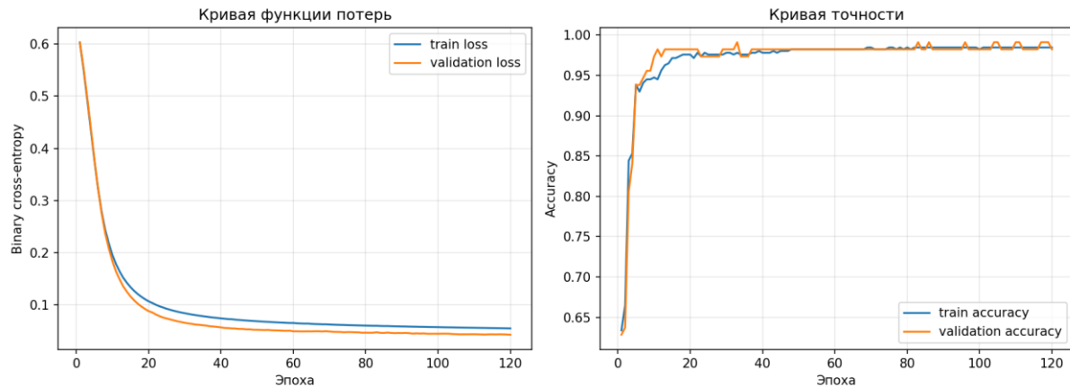
Рисунок 2 — Кривые функции потерь и точности
